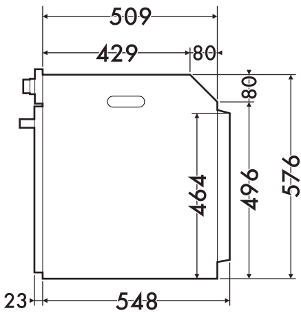
(вид сбоку)
